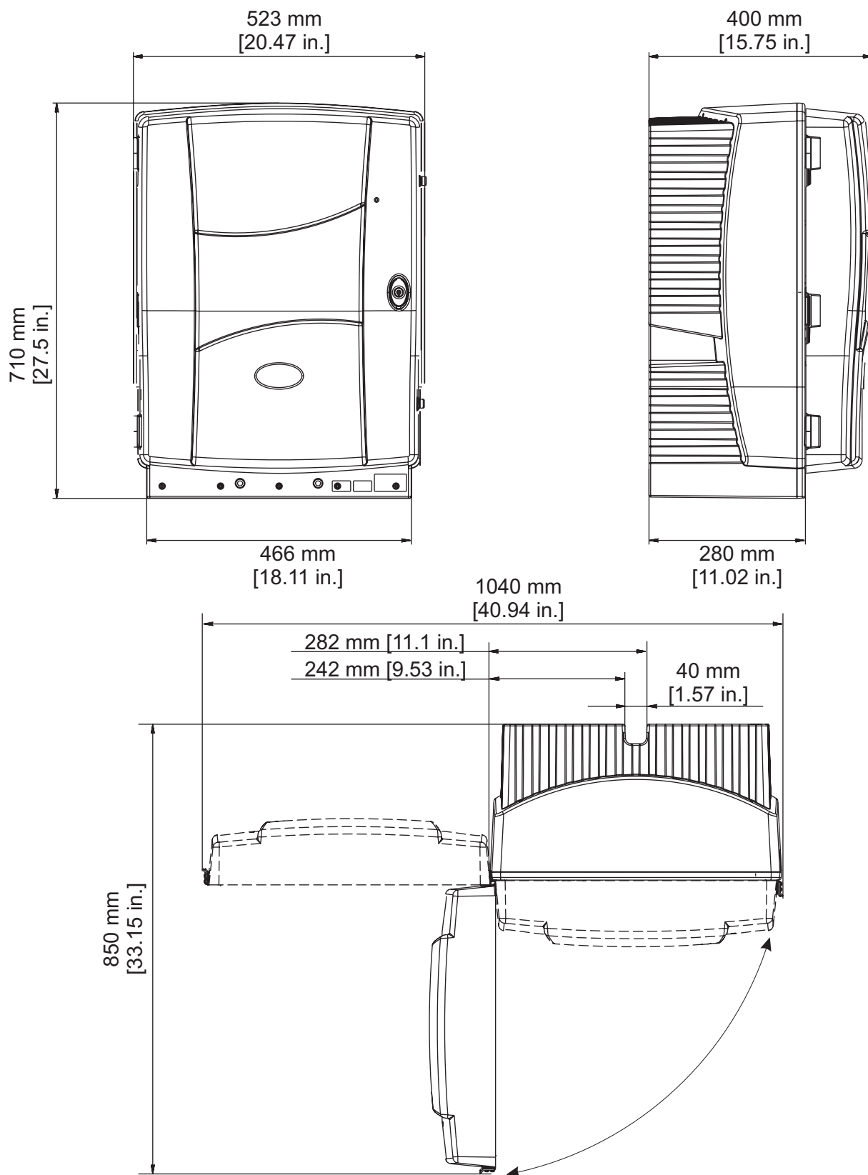
Figur 1 Måttritning
